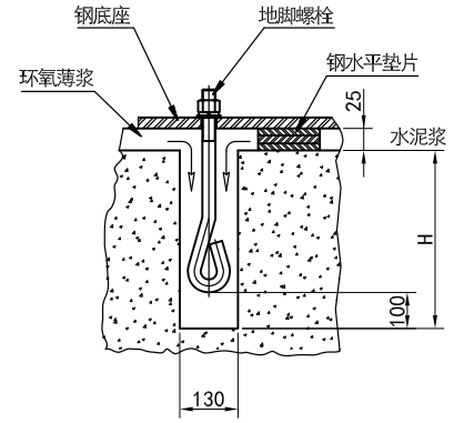
G-G地脚螺栓安装示意图 不按比例
